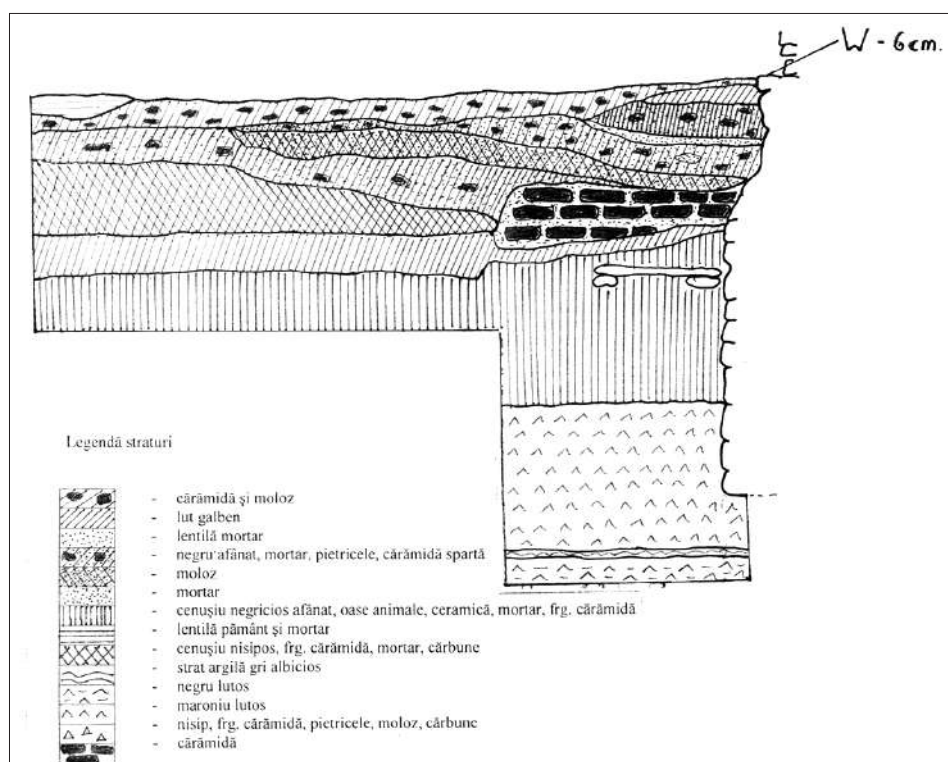
Fig. 7. Corp C3, S1, profil nordic, scara 1:20.
