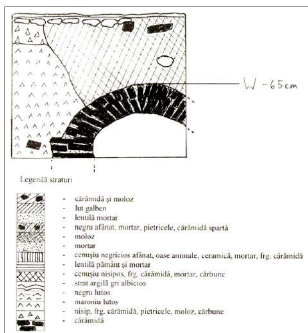
Fig. 12. Tronson 1 canalizare est-vest, Bolta 2, scara 1:20.
