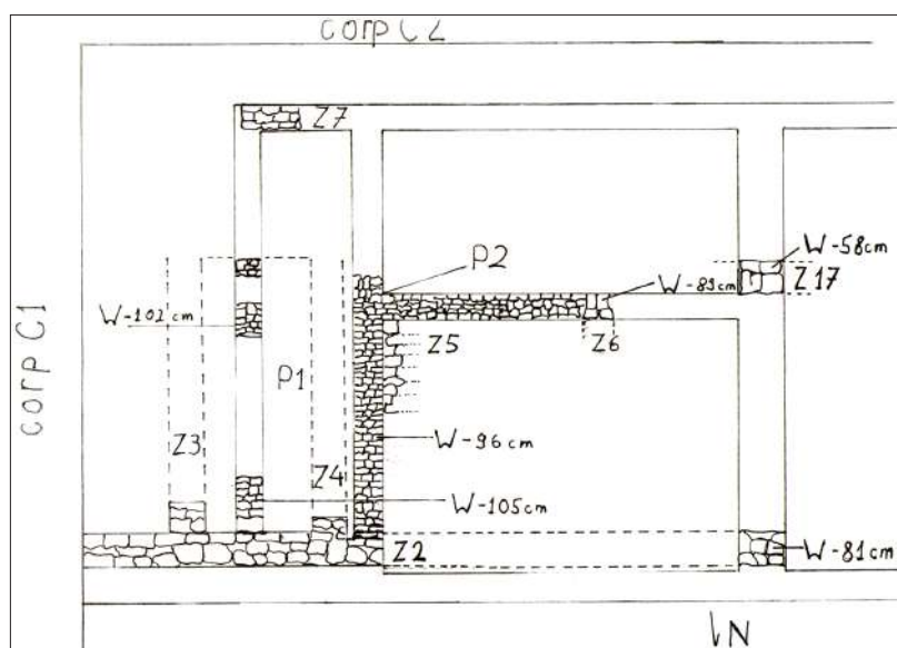
Fig. 18. Locuința L1, scara 1:75.
