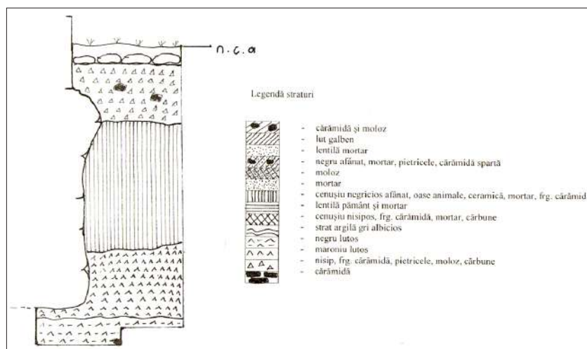
Fig. 8. Corp C3, S2, profil nordic, scara 1:20.
