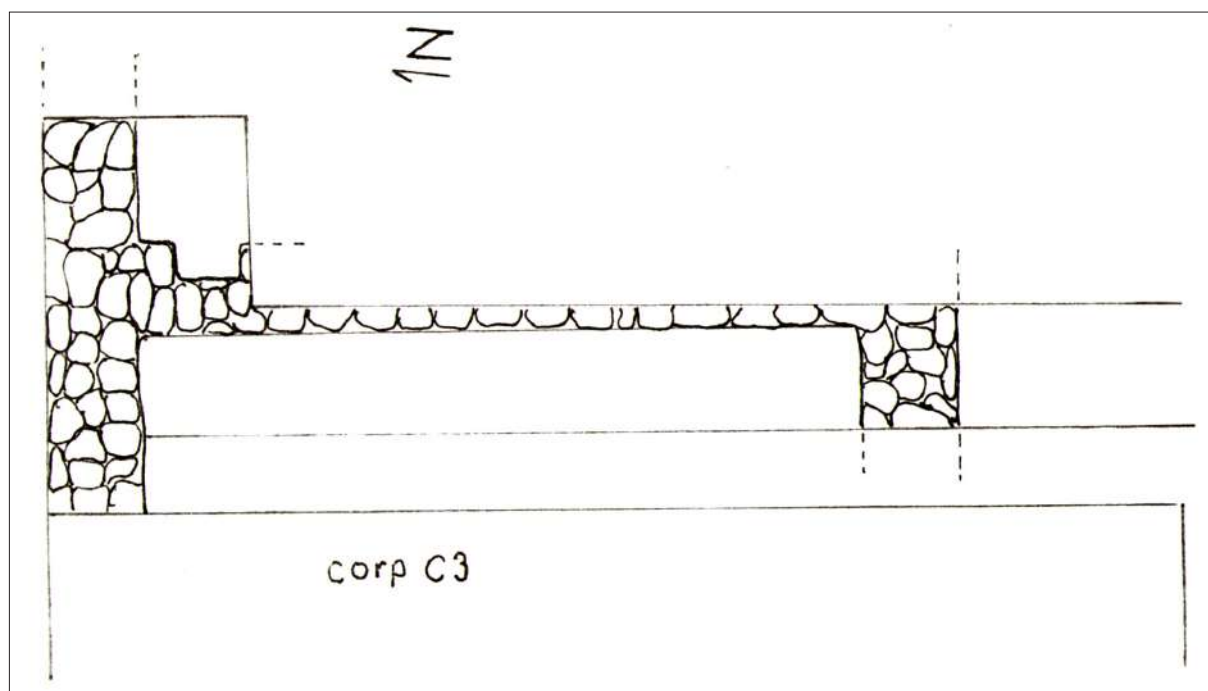
Fig. 30. Corp C3 parte demolată, detaliu tronson nordic, scara 1:50.
