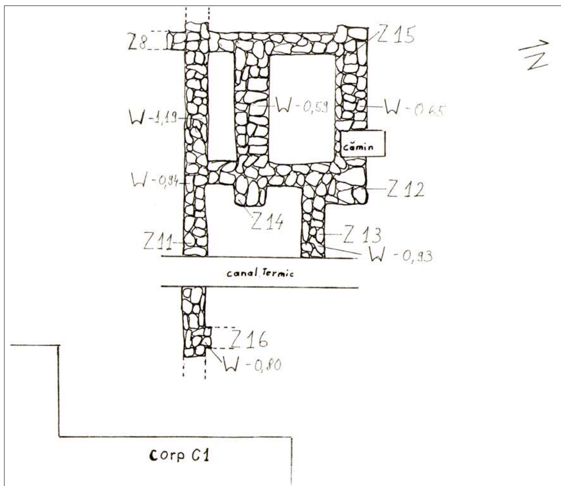
Fig. 29. Corp C3 parte demolată, detaliu turn, scara 1:75.
